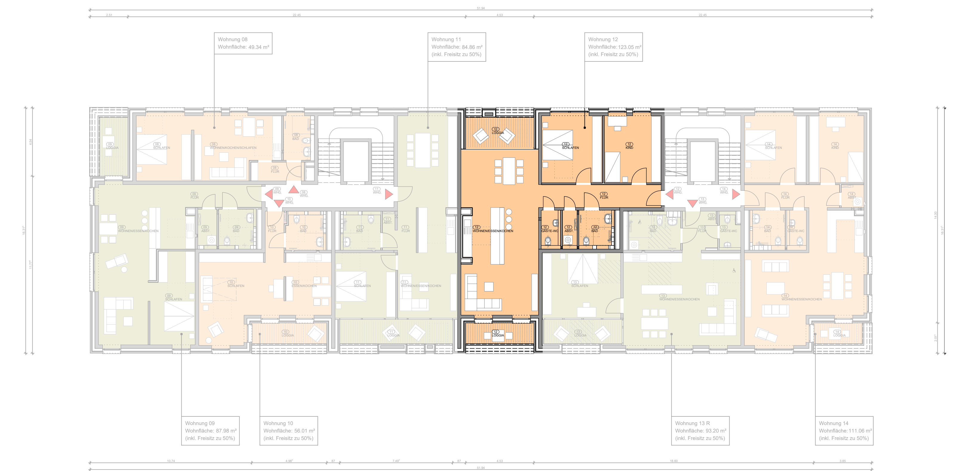
HAUS 1 - 1.OBERGESCHOSS
